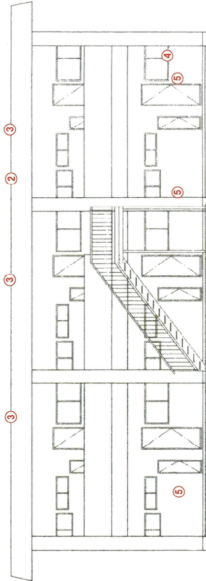
【北立面図】
