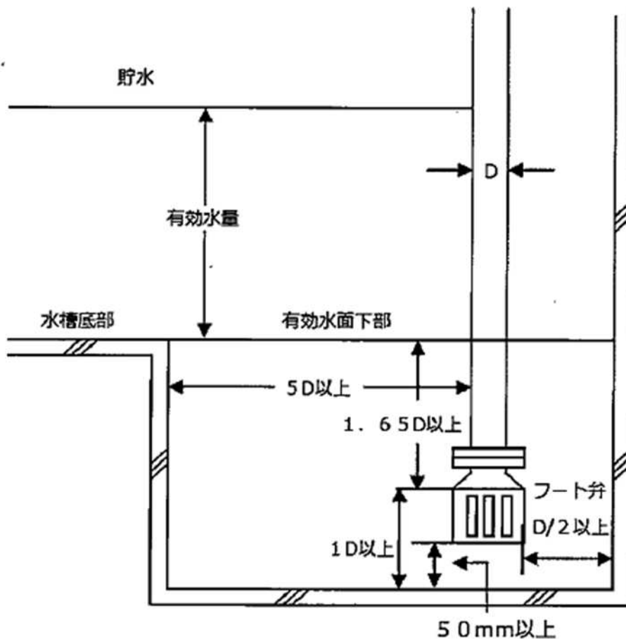
図2（サクシヨンピットを設ける場合）
