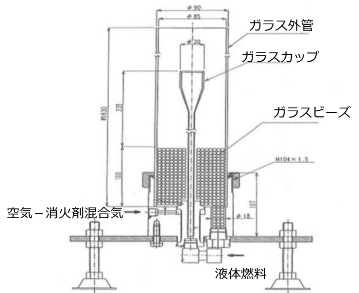
図2 カップ燃焼装置 (FRIガラスカップバーナー)
