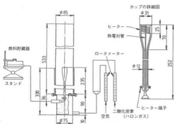
図1 カップ燃烧装置
