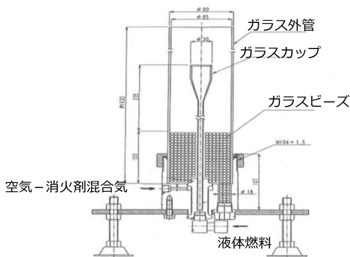
図2 カップ燃烧装置 (FRIガラスカップバーナー)
