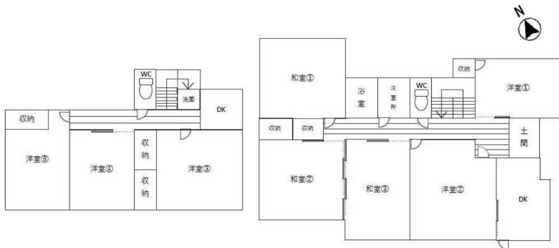
(2階) 平面図
