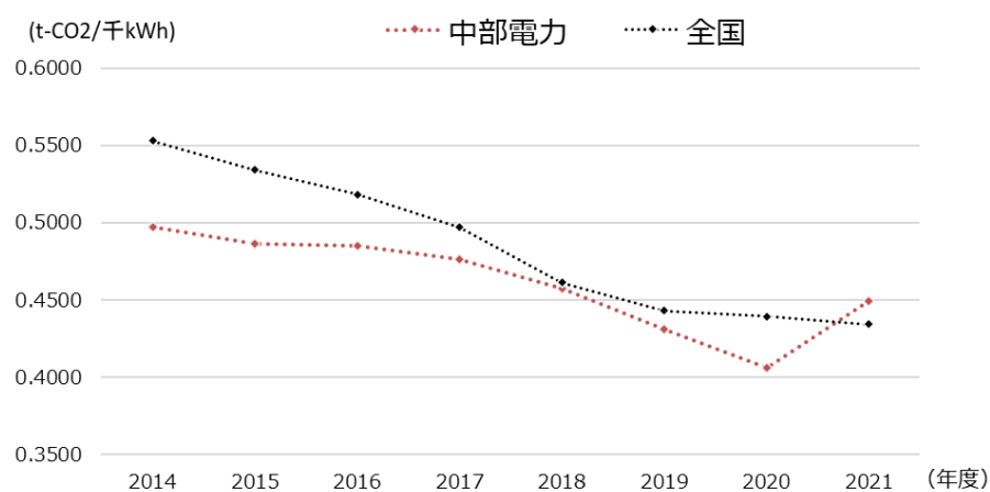
図 2-18 電力排出係数の推移
