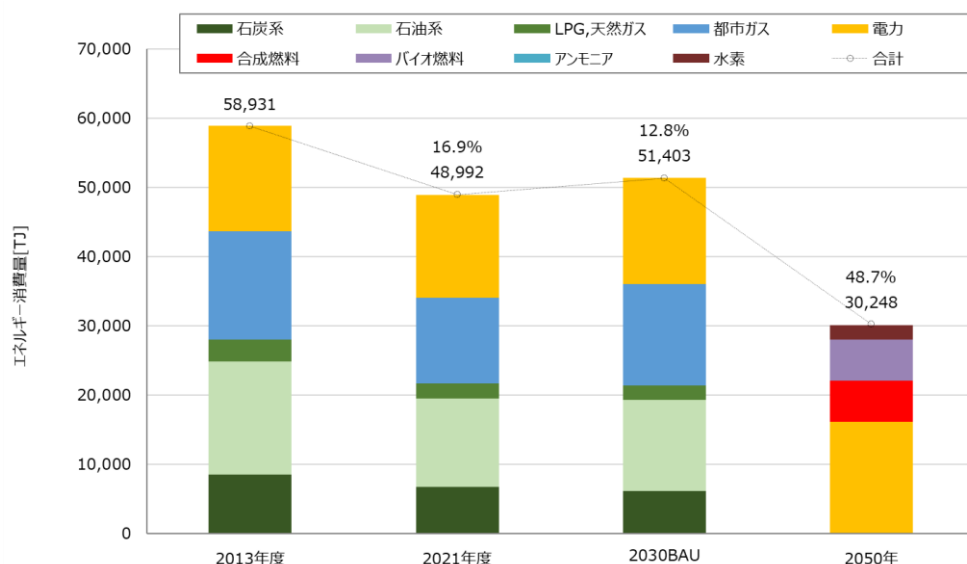
図 2-32 豊田市の 2050 年脱炭素シナリオ（エネルギー消費量）
