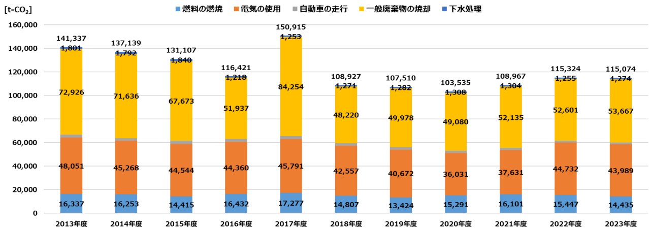
図 3-2 活動区分別の温室効果ガス排出量の推移
