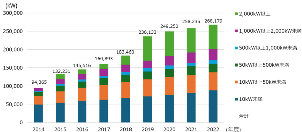
出典：再生可能エネルギー電気の利用の促進に関する特別措置法 情報公表用ウェブサイト（経済産業省）を基に作成 図 2-8 太陽光発電設備 FIT 導入容量の推移（発電容量別）
