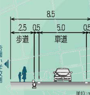
⑥ 市道 若林花園線
