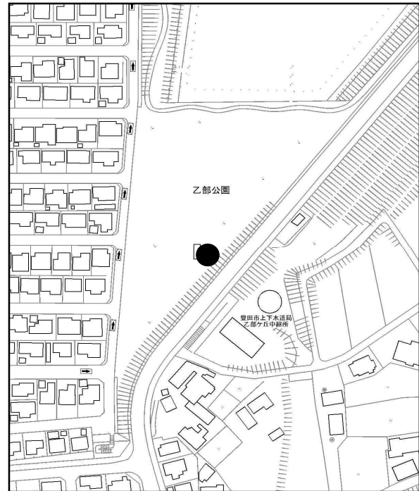
図4-2-11 環境騒音調査結果 (乙部ヶ丘)
