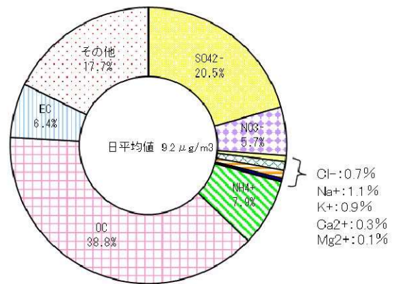
図1-10-2 各局の微小粒子状物質（PM2.5）成分分析 主要成分の割合
