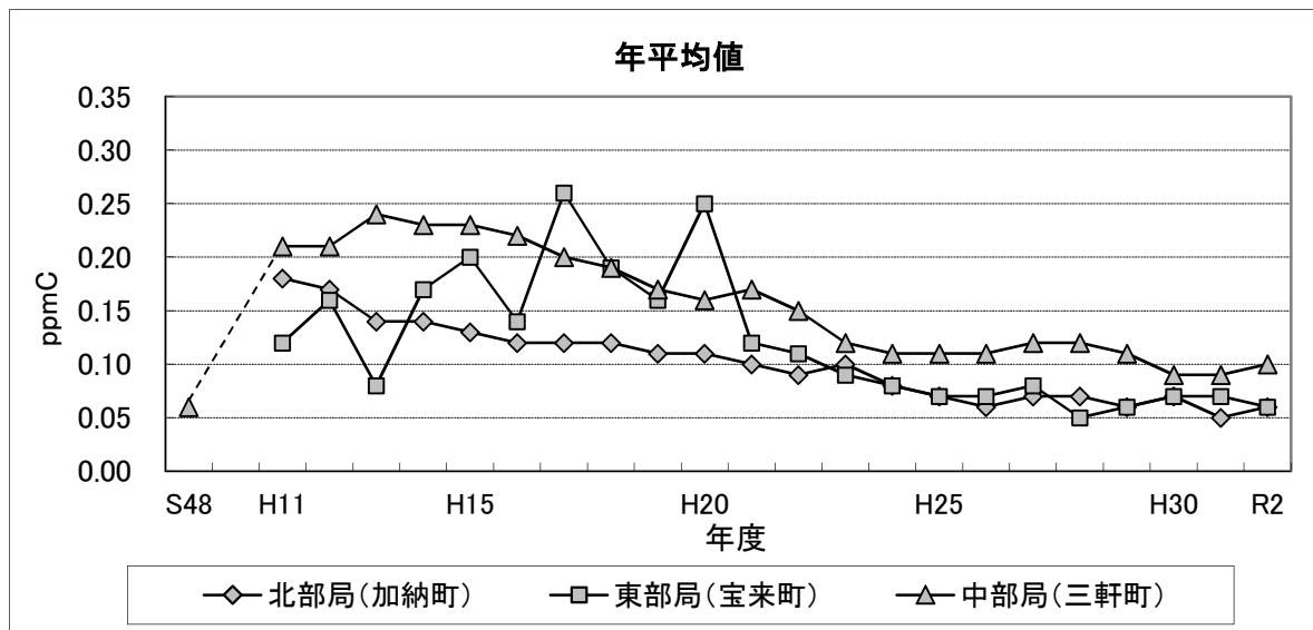
図1-9 非メタン系炭化水素の月別変化・経年変化
