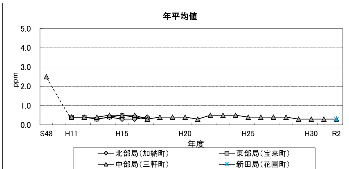
図 1-5 一酸化炭素の月別変化・経年変化
