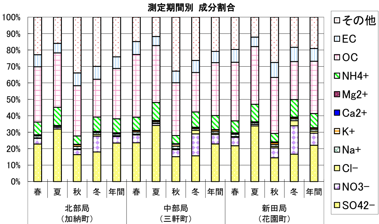
図 1-10-4 微小粒子状物質 成分量・割合
