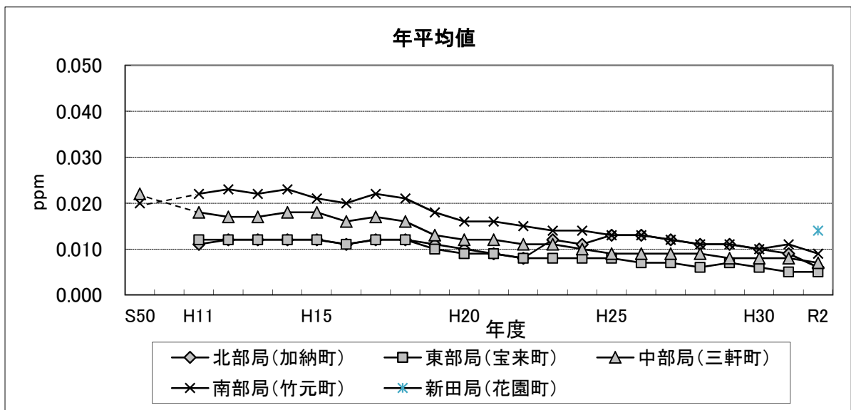
図 1-3 二酸化窒素の月別変化・経年変化
