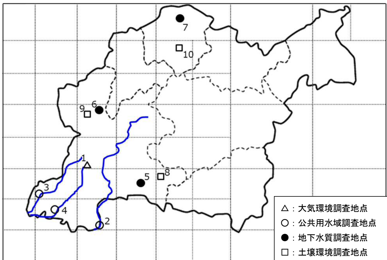
図 3-1 調査地点図
