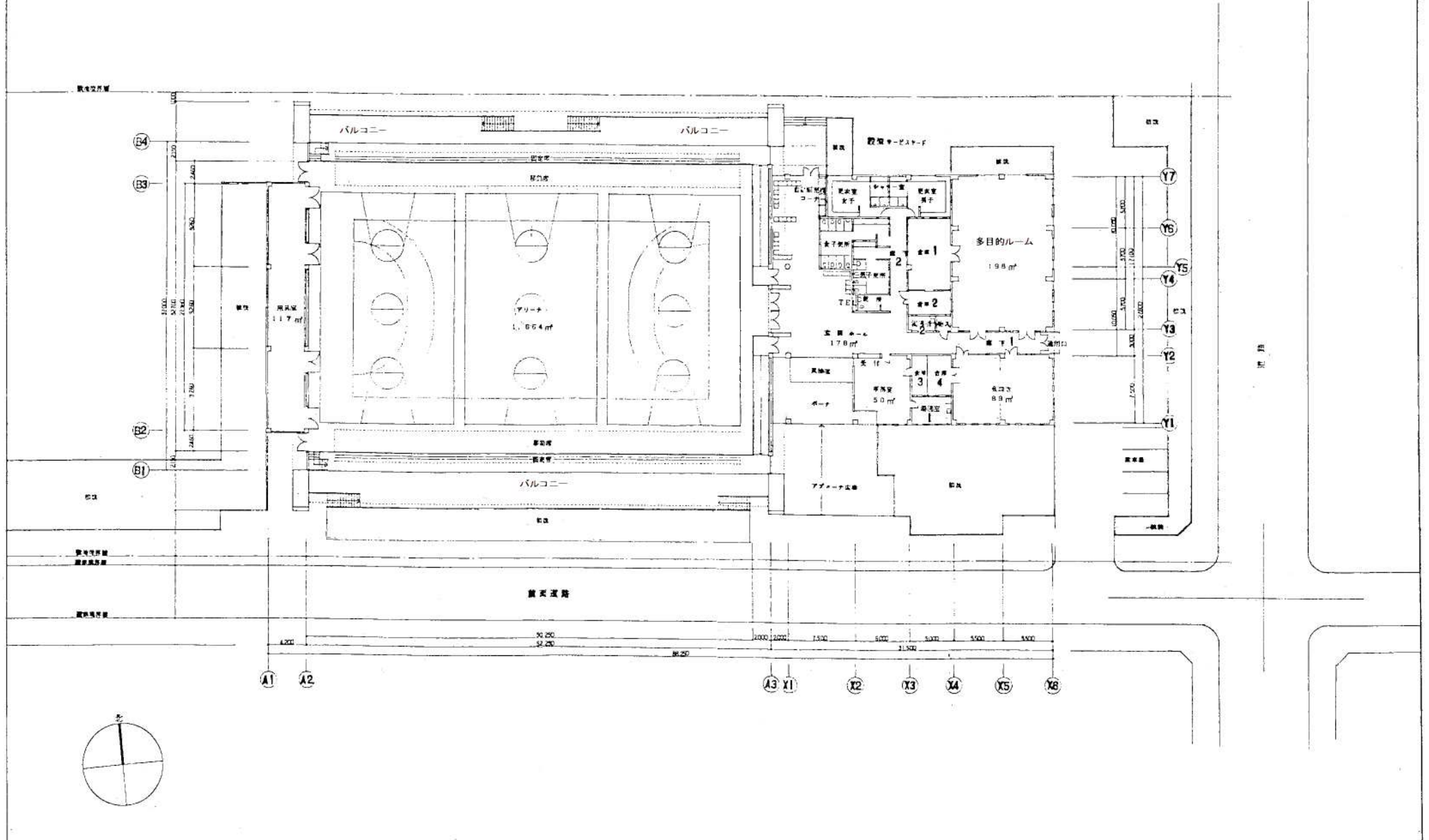
高岡公園体育館 配座・平面図
