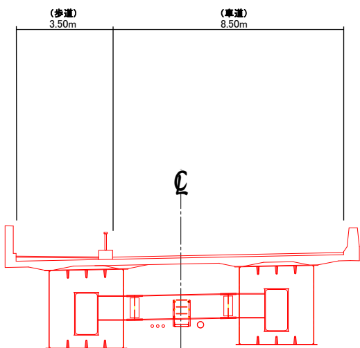
【渡河橋】断面図 (A-A)
