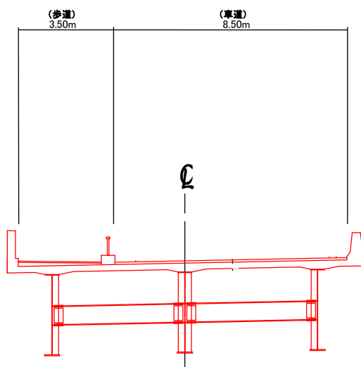
【高架橋】断面図 (B-B)
