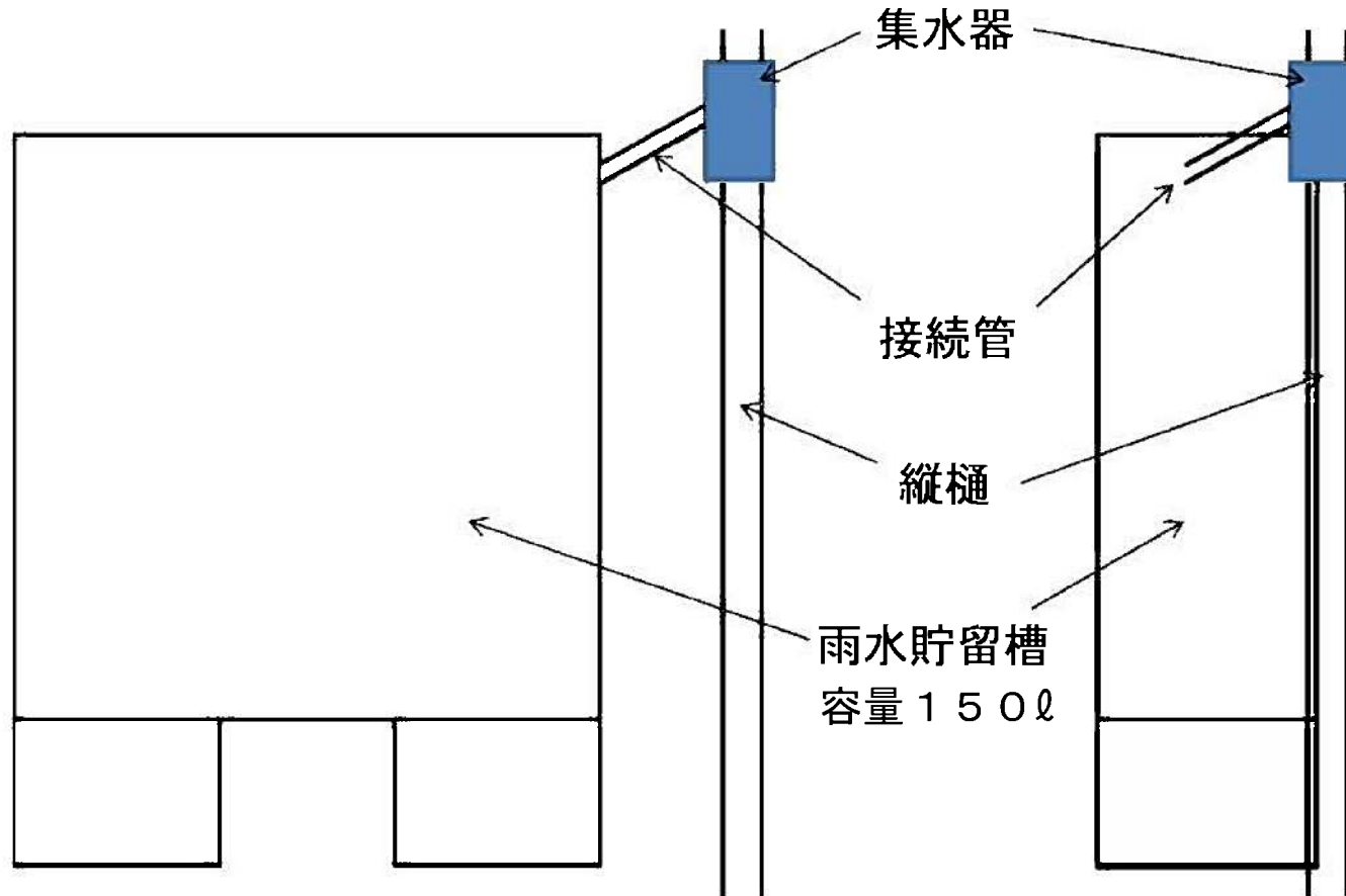
雨水貯留槽正面
