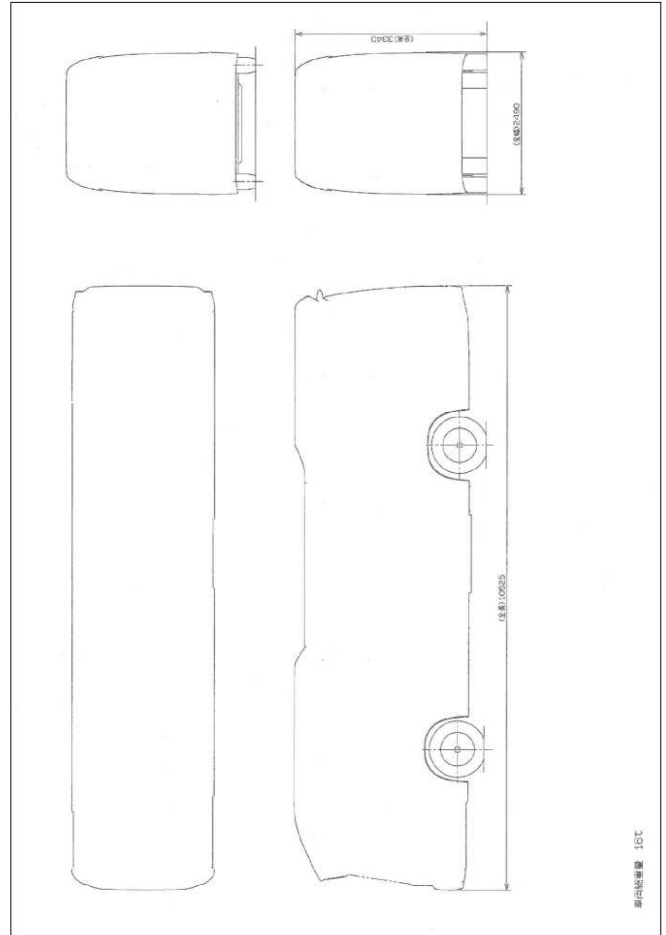
使用車両イメージ図（外観4面図）
