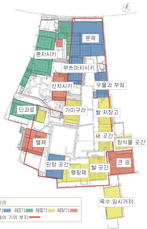
▲구 스즈키 가문 저택 평면도 (중문 16동)
