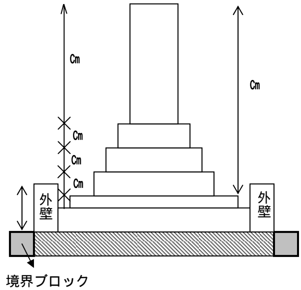
立面図
